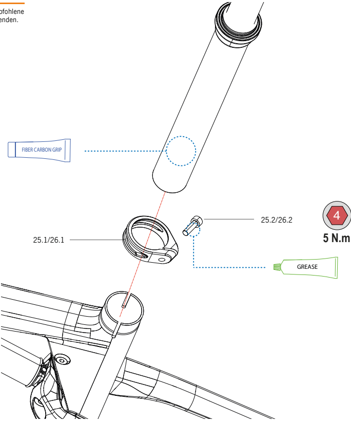
25 OIZ CARBON 23 SATTELSTÜTZENSCHELLE Titanschraube
